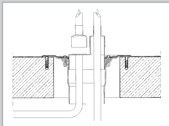
Przykład zastosowania MFD
