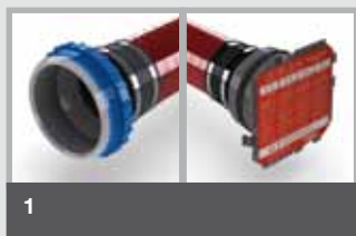
D / KB Pierwsza strona do połączenia ze szczelnym kołnierzem. Druga strona ze szczelnym kołnierzem do zabetonowania.
