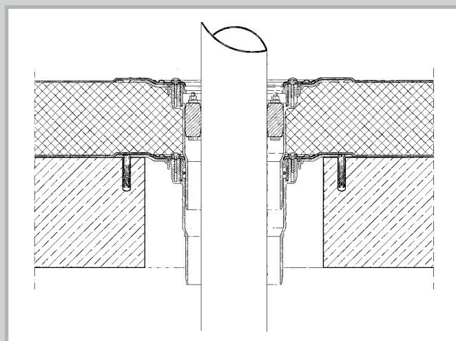
Przykład zastosowania MFD/AE (z podwójnym kołnierzem)
